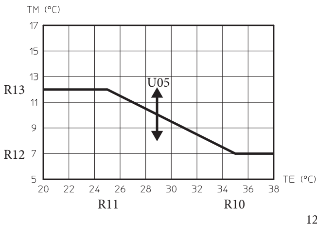
Θερμοκρασία κατάθλιψης στη ζώνη 1 σε φάση ψύξης και παρουσία εξωτερικού αισθητήρα
