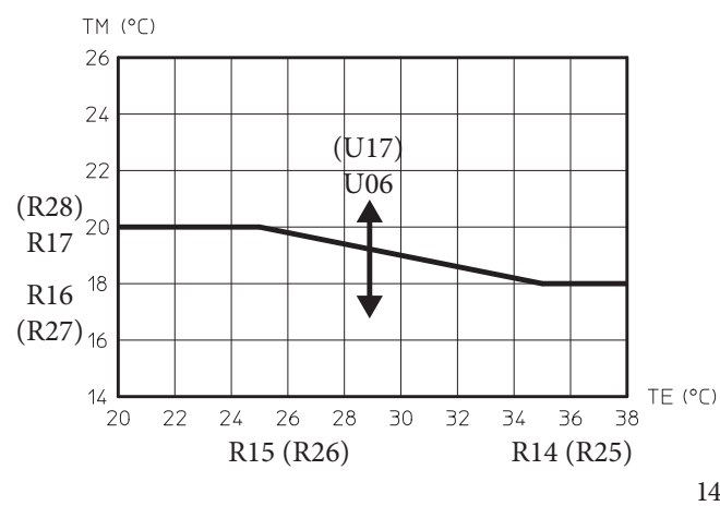
Θερμοκρασία κατάθλιψης στη μικτή ζώνη 2 (3) σε φάση ψύξης και παρουσία εξωτερικού αισθητήρα
