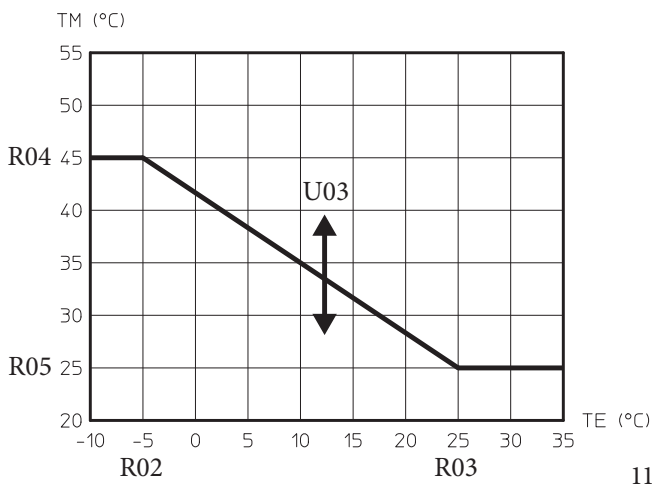
Θερμοκρασία κατάθλιψης στη ζώνη 1 σε φάση θέρμανσης και παρουσία εξωτερικού αισθητήρα
