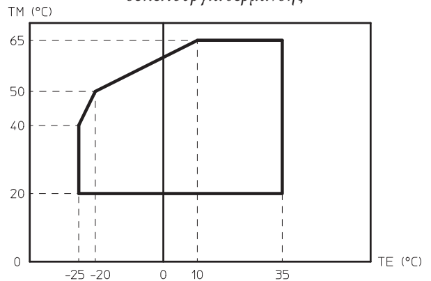
Όρια λειτουργίας της αντλίας θερμότητας σε λειτουργία θέρμανσης
