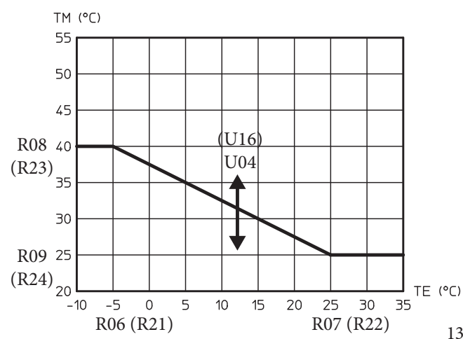
Θερμοκρασία κατάθλιψης στη μικτή ζώνη 2 (3) σε φάση θέρμανσης και παρουσία εξωτερικού αισθητήρα
