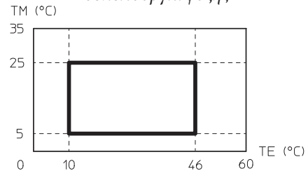
Όρια λειτουργίας της αντλίας θερμότητας σε λειτουργία ψύξης
